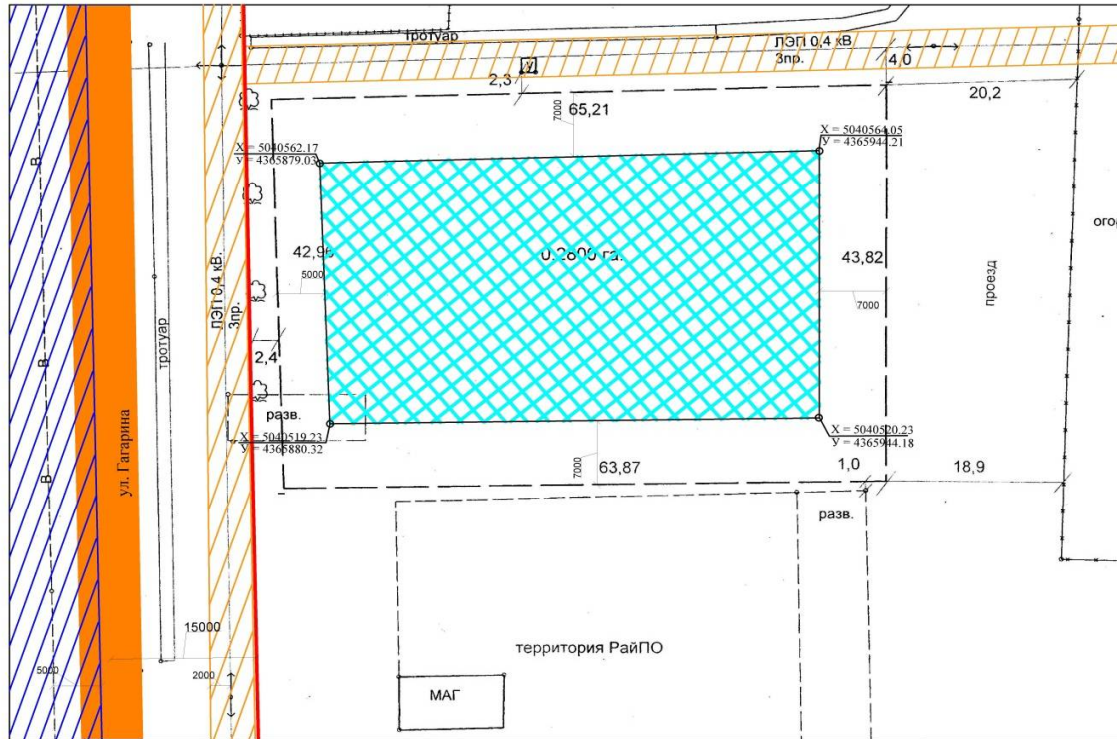
Чертеж градостроительного план земельного участка и линий градостроительного регулирования
